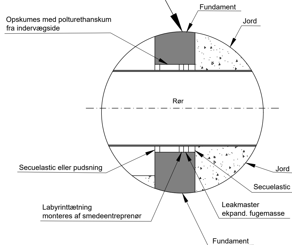
Gennemførings detalje
