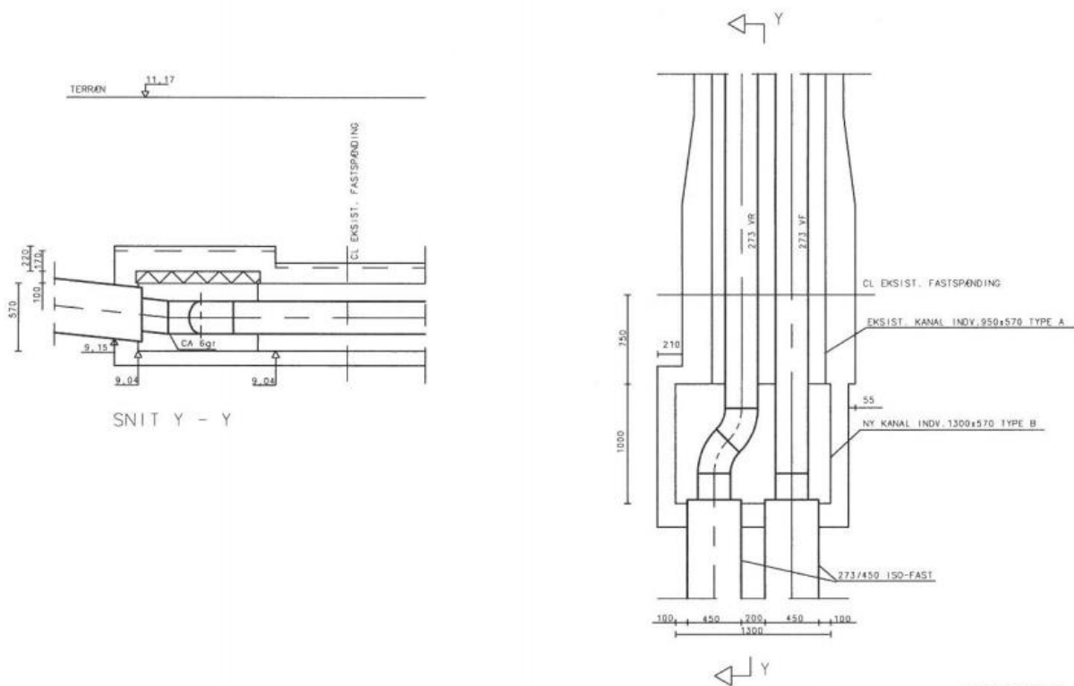
Figur 3 Videreføring med præisolerede stålør fra blind ende på betonkanal
