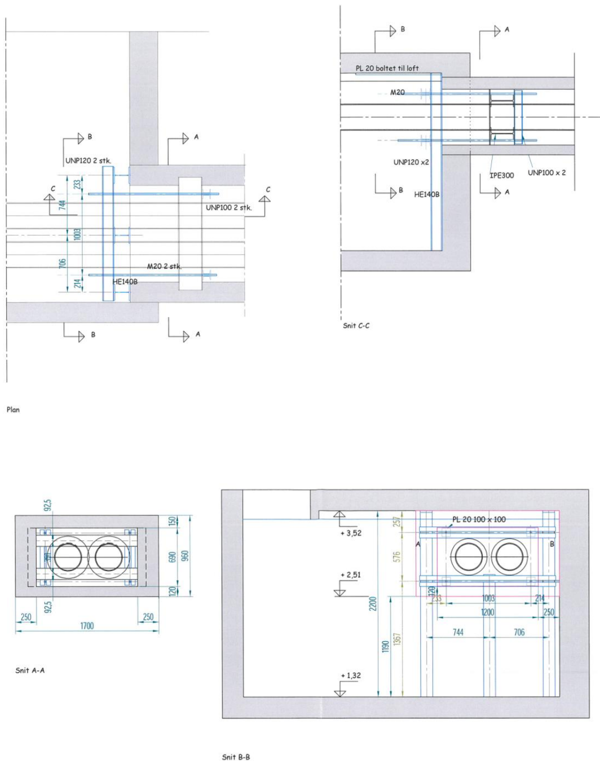
Figur 4 Eksempel på supplerende fastspænding i kammer
