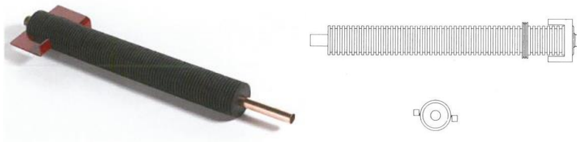
Figur 2 Væggennemføring med indstøbningsankre
