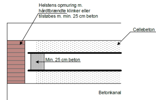
Figur 6.1 Type A – Længdesnit for kanal \leq 400 \times 500 mm
