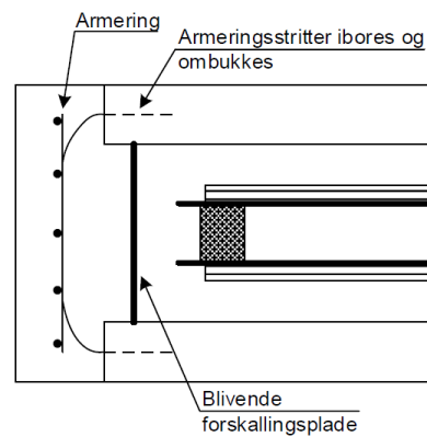
Figur 6.4 Type B – Længdesnit for kanal > 400 x 500 mm
