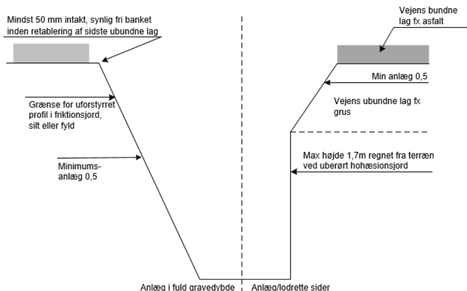
Figur 3.3 Graveprofil, uafstivet grav (udklip fra tegning 52-0737)
