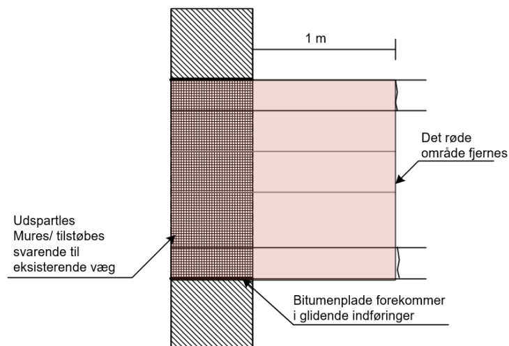
Figur 6.6 Nedlægning af betonkanalindføring
