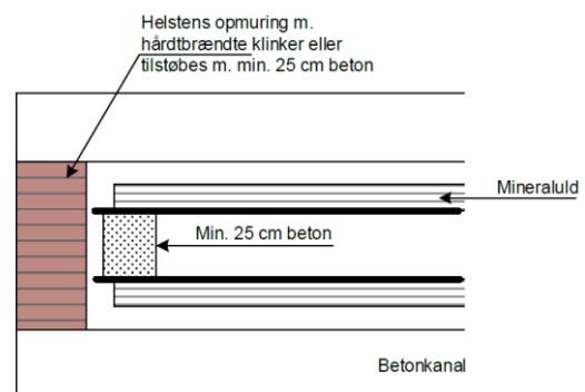
Figur 6.2 Type B- Længdesnit for kanal \leq 400 \times 500
