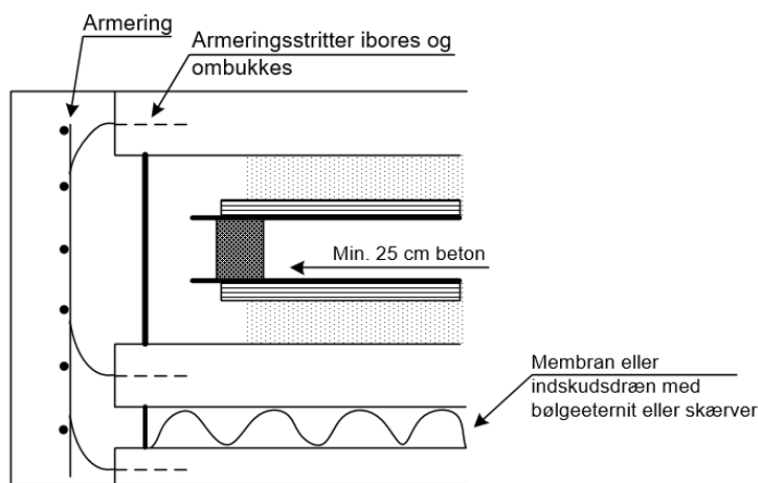
Figur 6.5 Type C og D - Længdesnit
