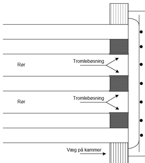
Figur 6.7 Lodret snit
