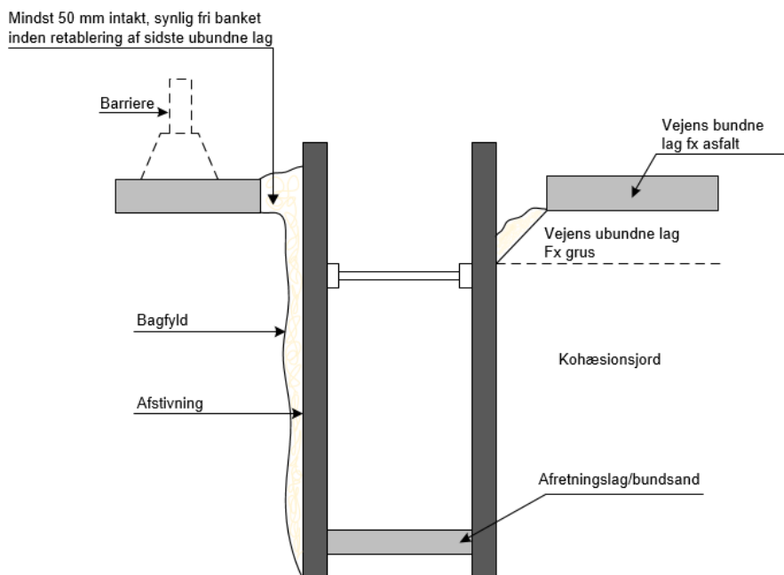
Figur 3.1 Graveprofil, afstivet grav (udklip fra tegning 52-0737)
