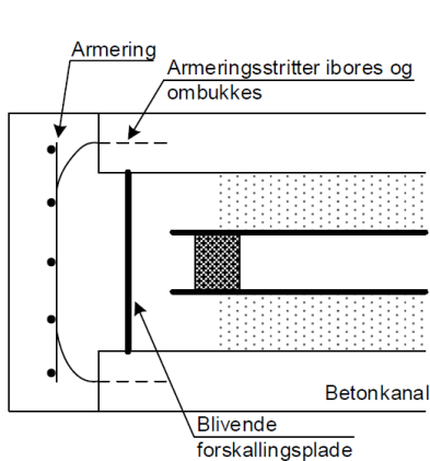
Figur 6.3 Type A – Længdesnit for kanal > 400 x 500 mm
