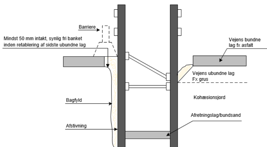
Figur 3.2 Graveprofil, afstivet grav med ekstra spænd (udklip fra tegning 52-0737)
