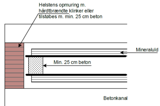
Figur 6.4 Type B – Længdesnit for kanal > 400 x 500
