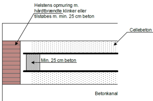
Figur 6.1 A – Længdesnit for kanal \leq 400 \times 500 mm
