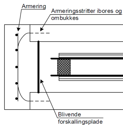
Figur 6.2 Type B- Længdesnit for kanal \leq 400 \times 500
