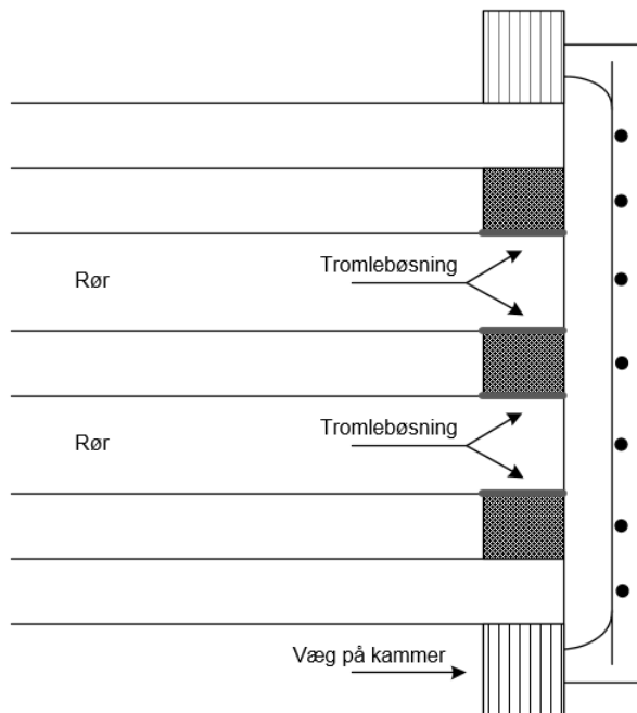
Figur 6.7 Lodret snit
