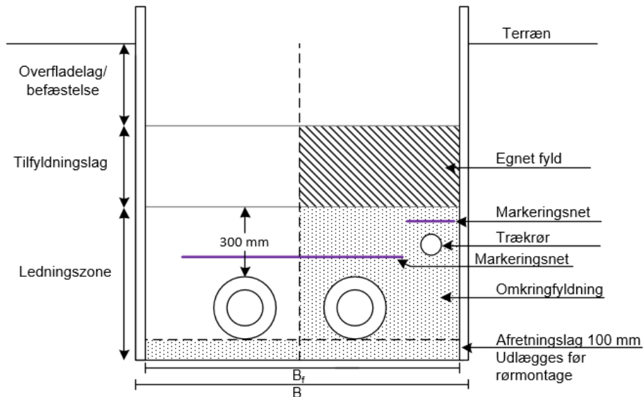
Figur 4.1 Tværsnit af ledningsgrav med præisolerede stålør (udklip fra tegning 52-0839)
