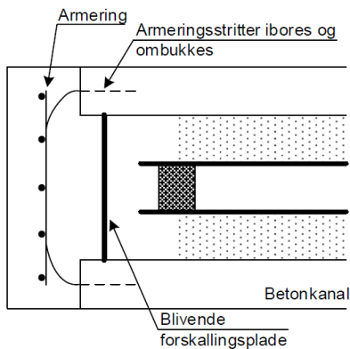
Figur 6.3 Type A – Længdesnit for kanal > 400 x 500 mm
