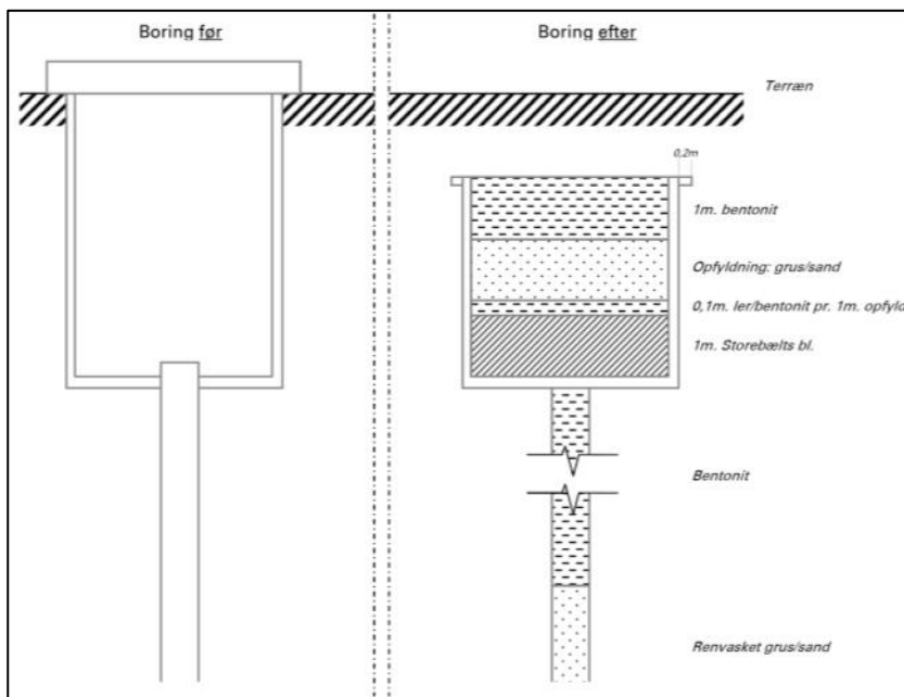
Figur 1 Principskitse i forhold til sløjfning af indvindingsboringer i brønd.
