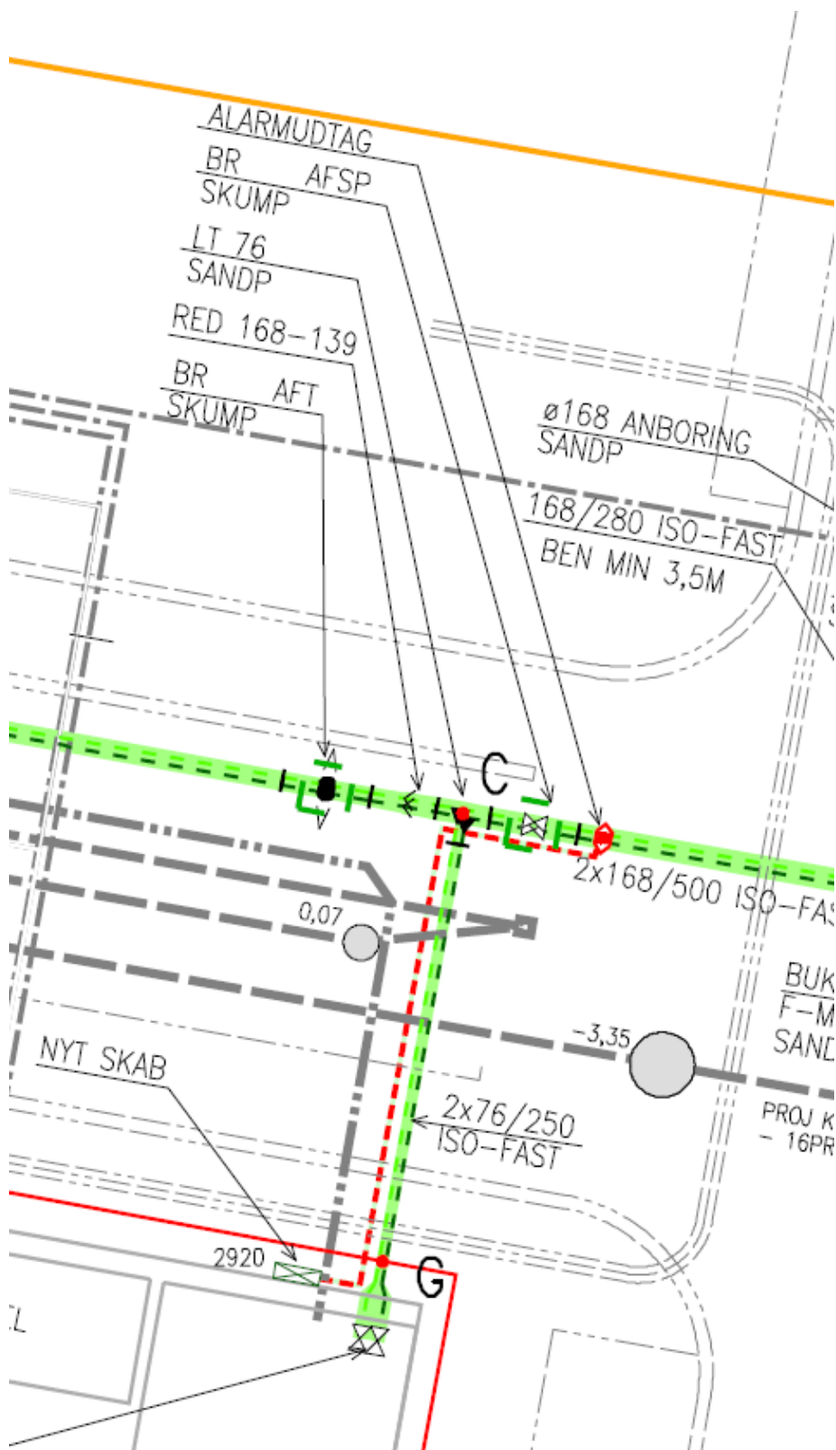
Figur 1 Udsnit af ledningsplan
