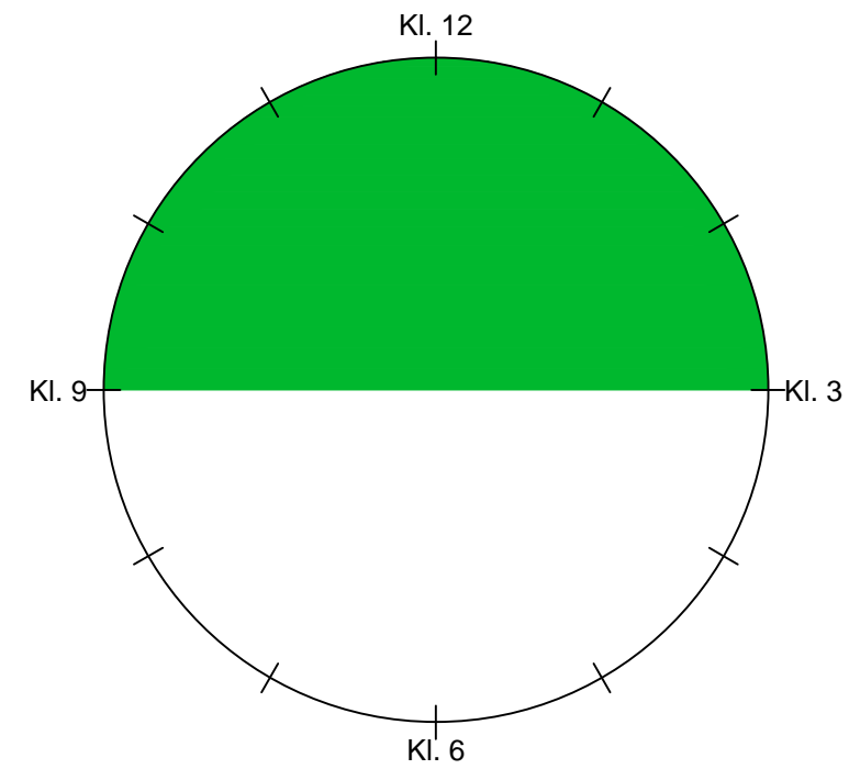
Placering af trækrør i ledningstværsnit over ø800mm
