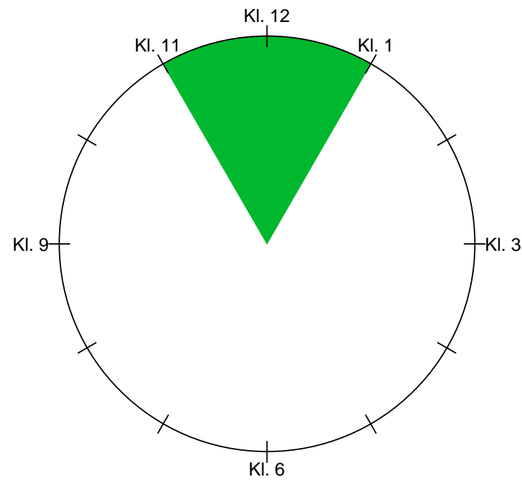
Placering af trækrør i ledningstværsnit under ø800mm
