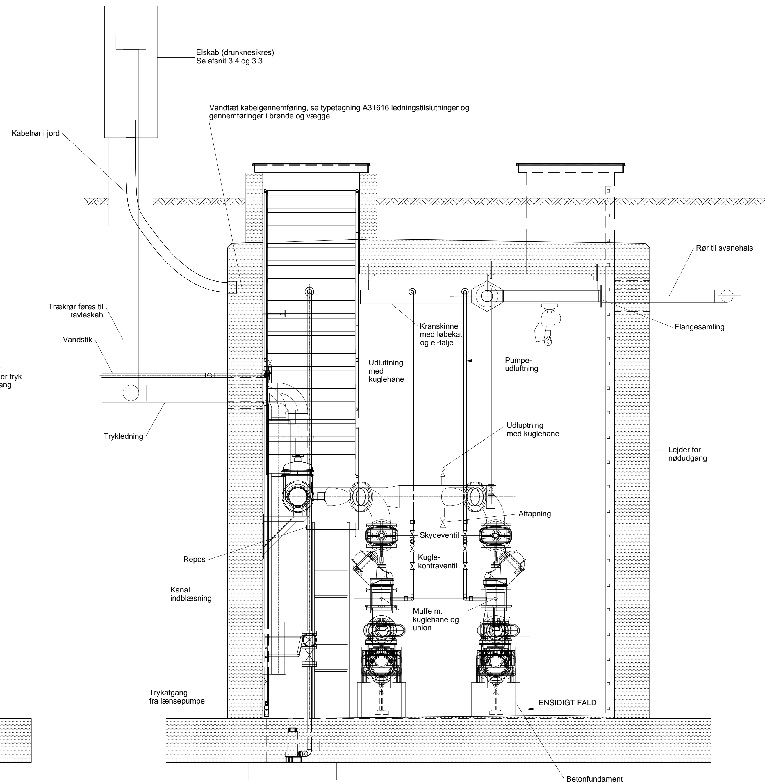
Snit D-D, 1:25
